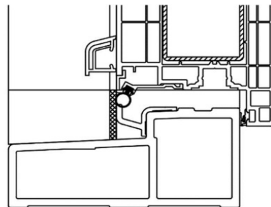
Afbeelding 8: Dubbele dichting
